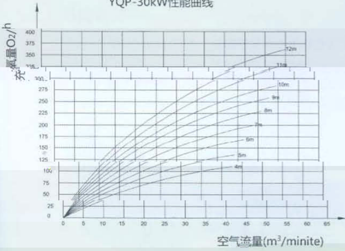
YQP-30kW性能曲线
